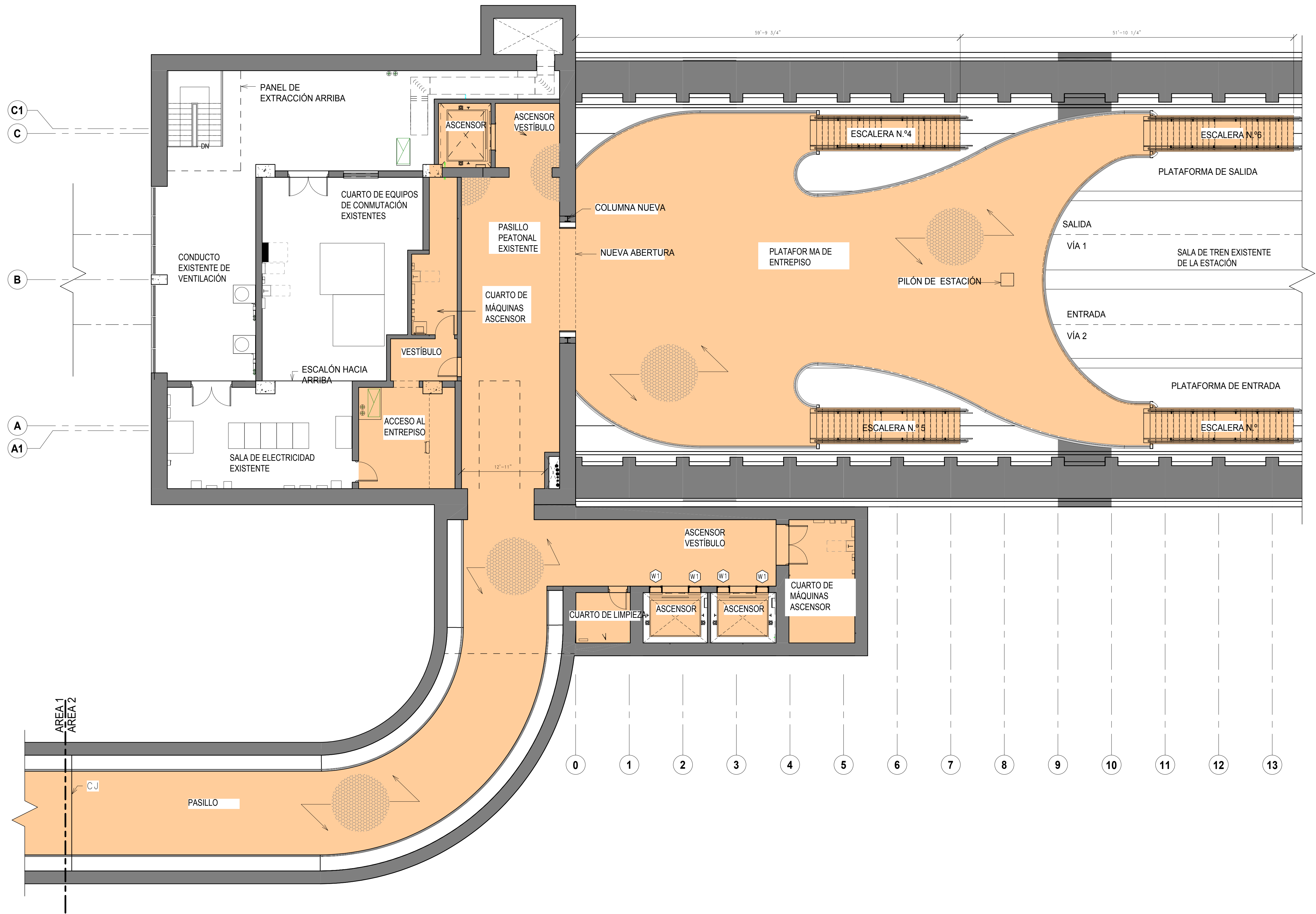
1 PLANO DE PLANTA: NIVEL ENTREPISO: ÁREA 2 1/8" = 1'-0"
