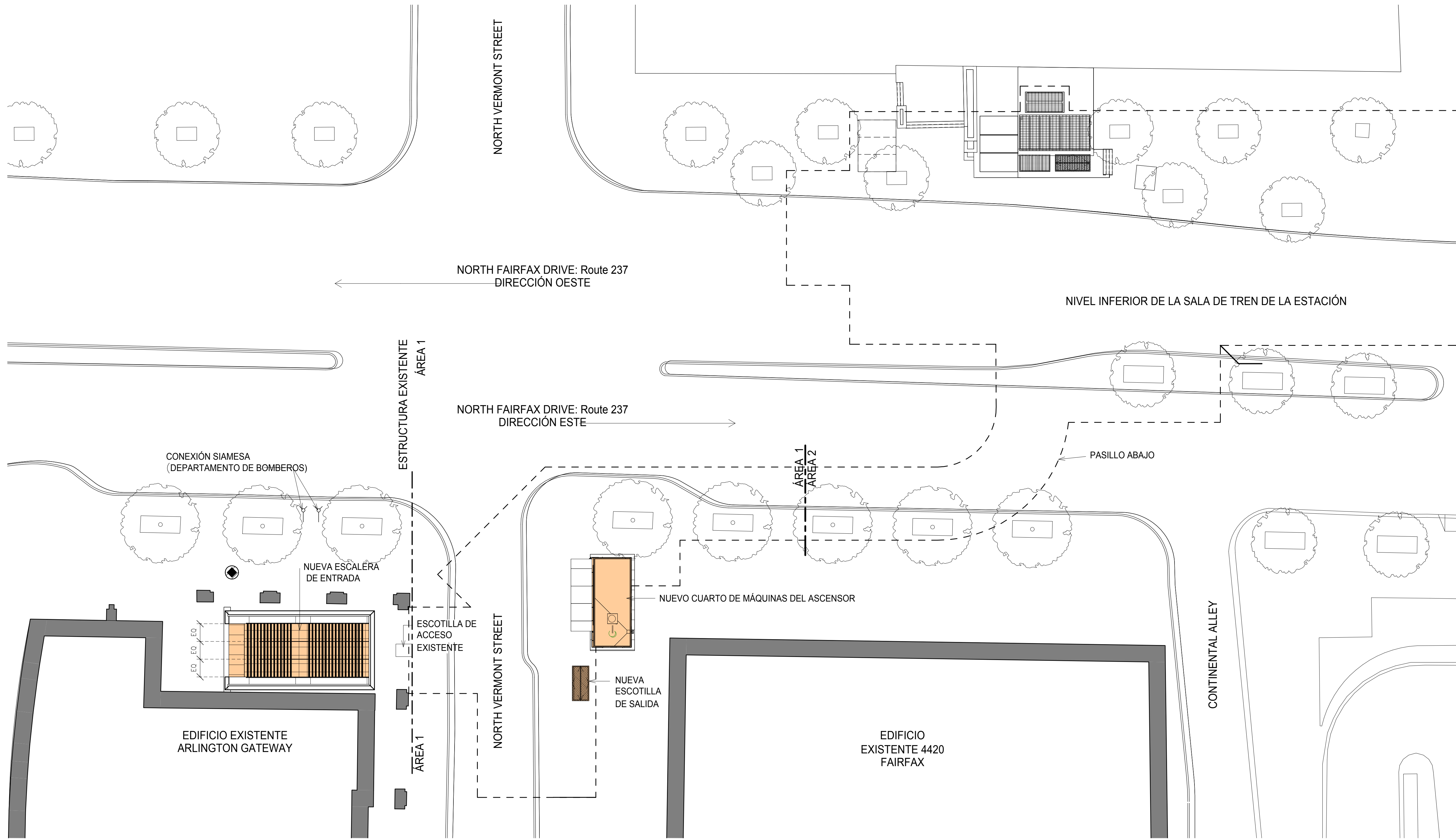
PLANO DEL SITIO
