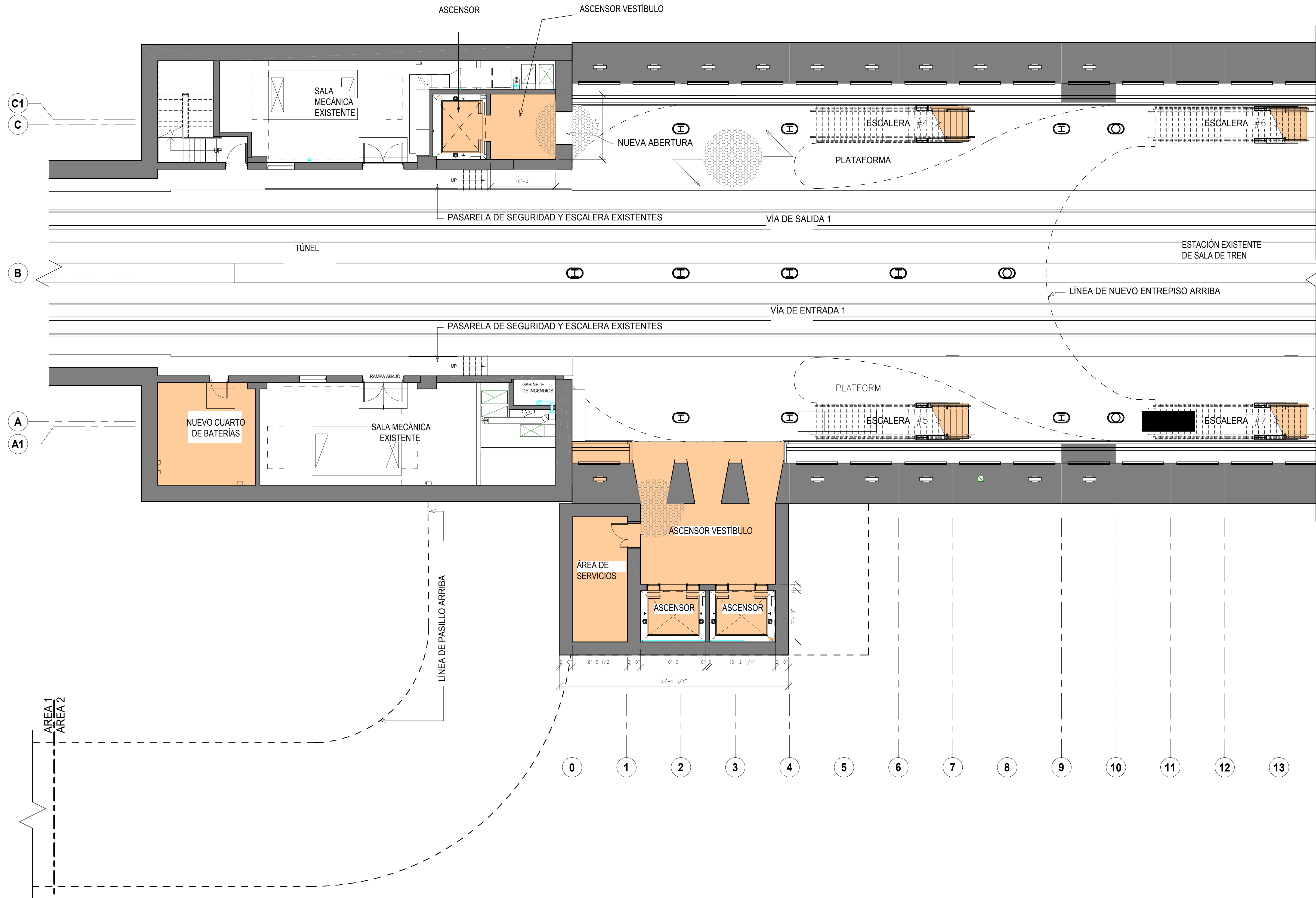
1 PLANO DE PLANTA: NIVEL DE PLATAFORMA 8 1/8" = 1'-0"
